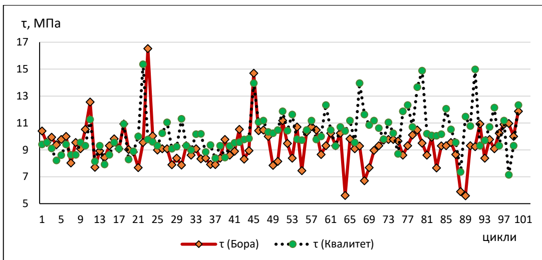
Рис. 3.4. Кінетика зміни напруження зсуву мастильного шару в контакті ( \tau ).
