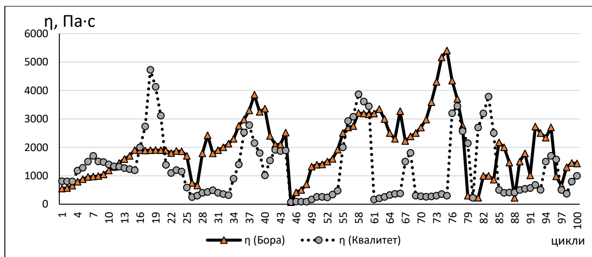
Рис. 4.5. Кінетика зміни ефективної в'язкості оливи ( \eta ) в контактї.
