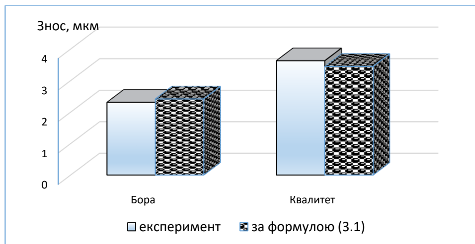
Рис. 3.9. Загальний лінійний знос випереджаючої та відстаючої поверхонь при змащуванні гідравлічною оливою АМГ-10 виробників Бора та Квалитет.
