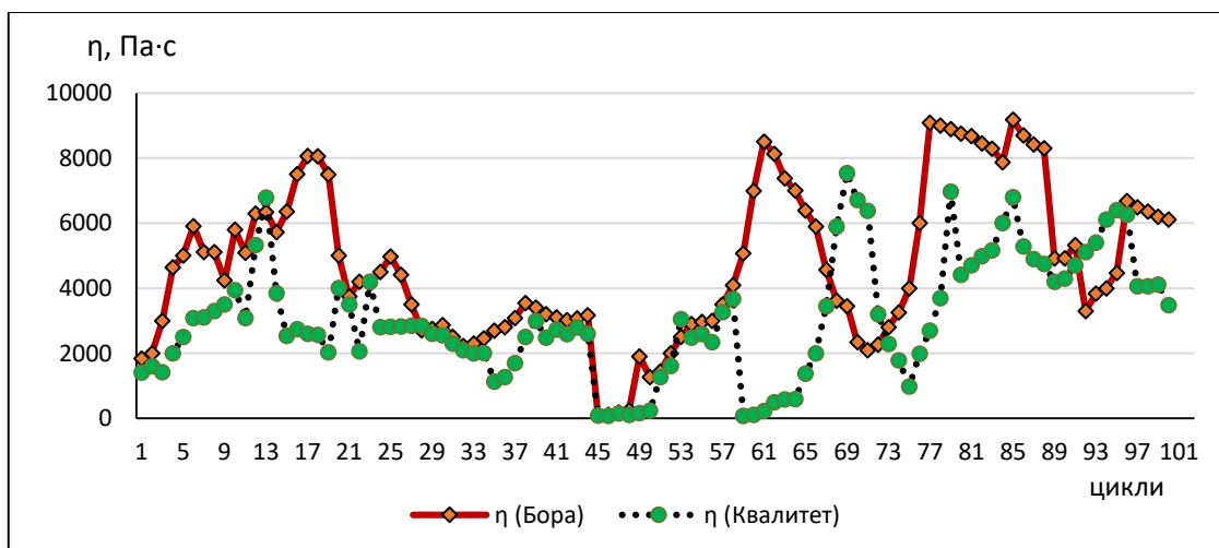
Рис. 3.5. Кінетика зміни ефективної в'язкості оливи ( \eta ) в контакті.
