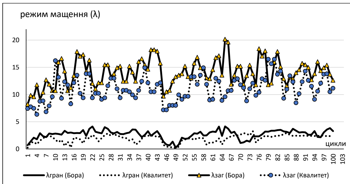
Рис. 3.3. Кінетика зміни режиму мащення в триботехнічному контактї.
