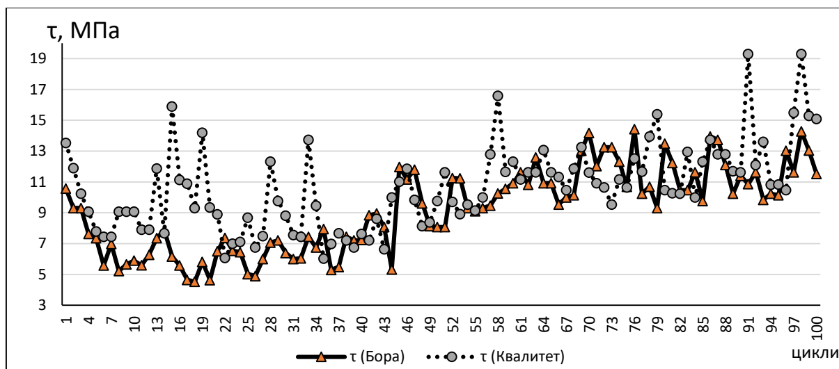
Рис. 4.4. Кінетика зміни напруження зсуву мастильного шару в контактї ( \tau ).
