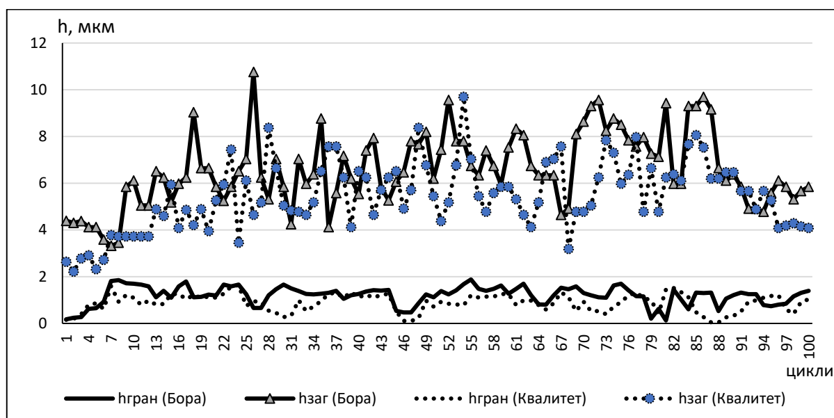
Рис. 4.2. Формування граничних адсорбційних шарів ( h_{\text{гран}} ) та загальної товщини мастильного шару ( h_{\text{заг}} ) в фрикційному контакті при напруженні.
