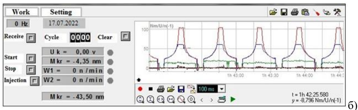
Рис. 2.3. Схема роботи двигунів установки тертя (а) та інтерфейс підпрограми обробки даних (б) при роботі трибосистеми в нестационарних умовах.
