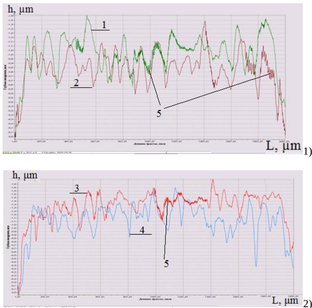
Рис. 4.9. Глибина вдавлення індентора при склерометрії: змащування зразком № 1 – випереджаюча (1) та відстаюча (2) поверхні, змащування зразком № 2 – випереджаюча (3) та відстаюча (4) поверхні, 5 – ділянки неоднорідного деформаційного мікрорельєфу.
