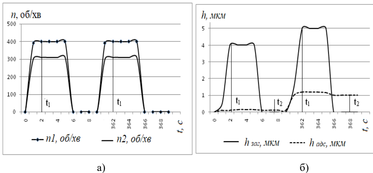
Рис. 2.7. Залежність частоти обертання дослідних зразків (а) та загальної товщини мастильного шару і товщини граничних шарів мастильного матеріалу (б) від часу роботи трибосистеми.
