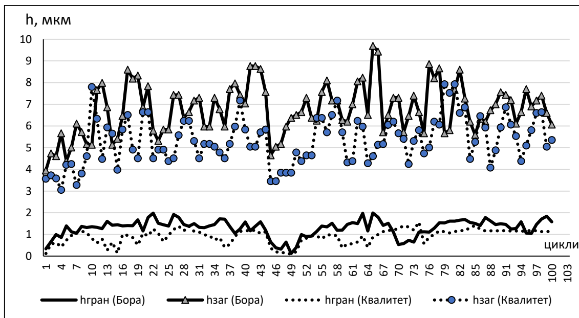
Рис. 3.2. Кінетика зміни товщини граничних адсорбційних шарів ( h_{\text{гран}} ) та загальної товщини мастильного шару ( h_{\text{заг}} ) в контактї при напрацюванні.
