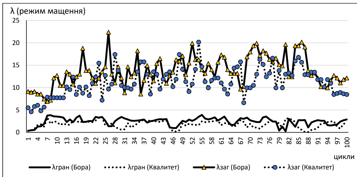
Рис. 4.3. Кінетика зміни режиму мащення в триботехнічному контакті: \lambda = 0 \dots 1 – домінування режиму без мастильного матеріалу; \lambda = 1 \dots 1,5 граничний; \lambda = 1,5 \dots 3 – змішаний; \lambda = 3 \dots 4 – еластогідродинамічний (контактно-гідродинамічний); \lambda \geq 4 – гідродинамічний.
